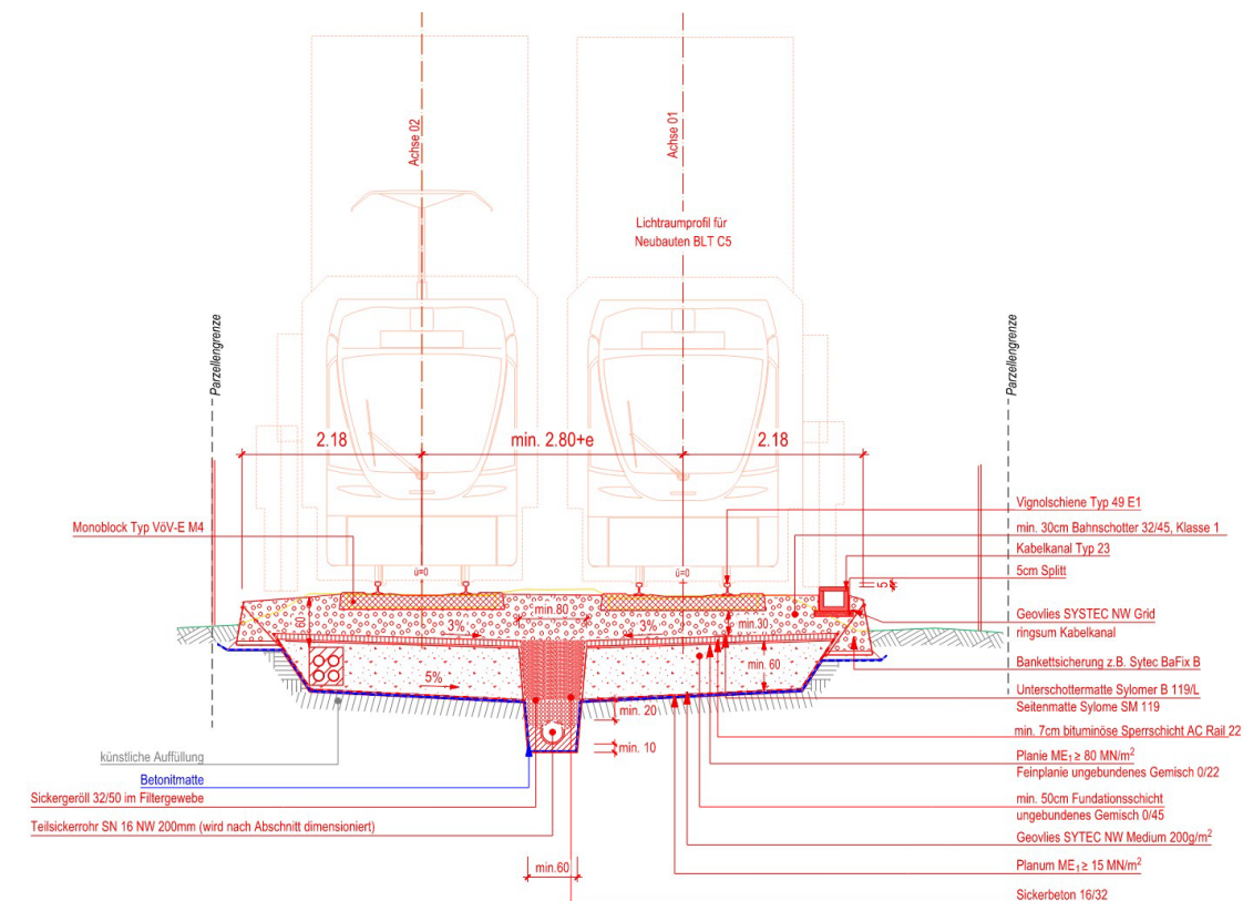
Schottergleis
