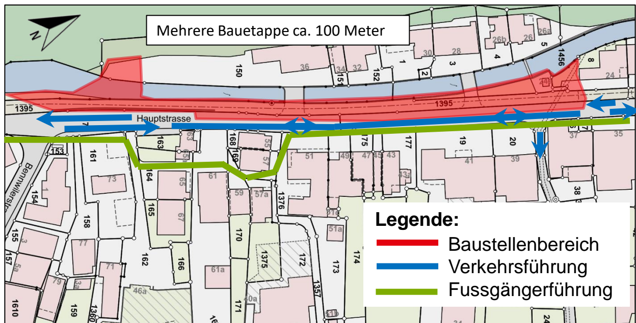
Skizze 1: Baustellenbereich Bachmauer A-07
